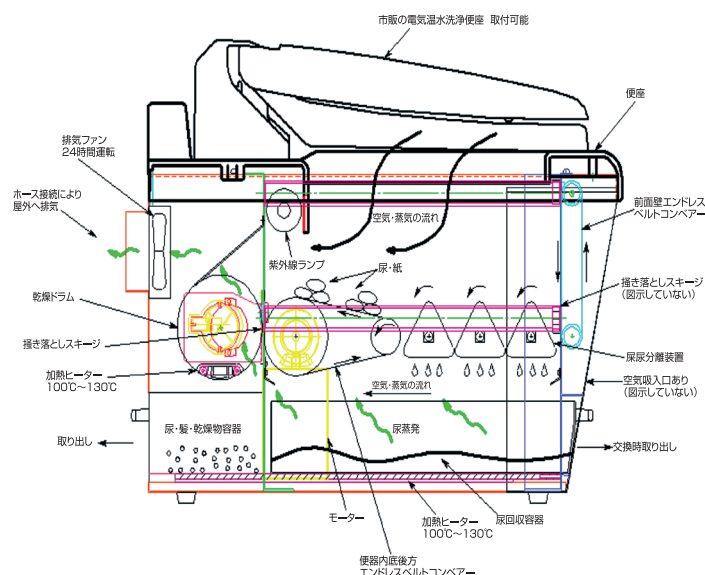
無水式乾燥し尿トイレ (横断面図)
